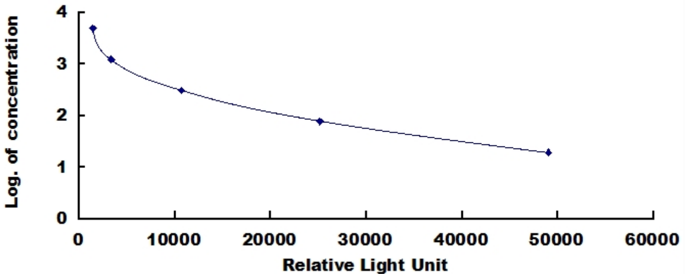
乙酰肉毒碱 (ALCAR) 检测试剂盒标准曲线
