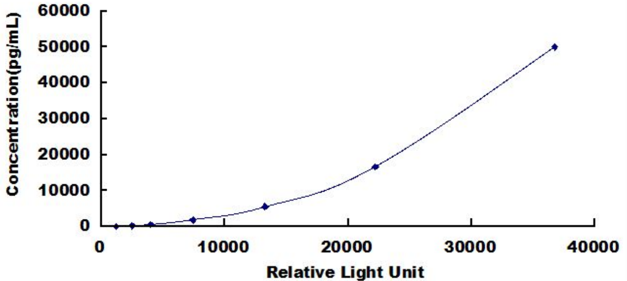
牛碱性磷酸酶 (ALP) 检测试剂盒标准曲线
