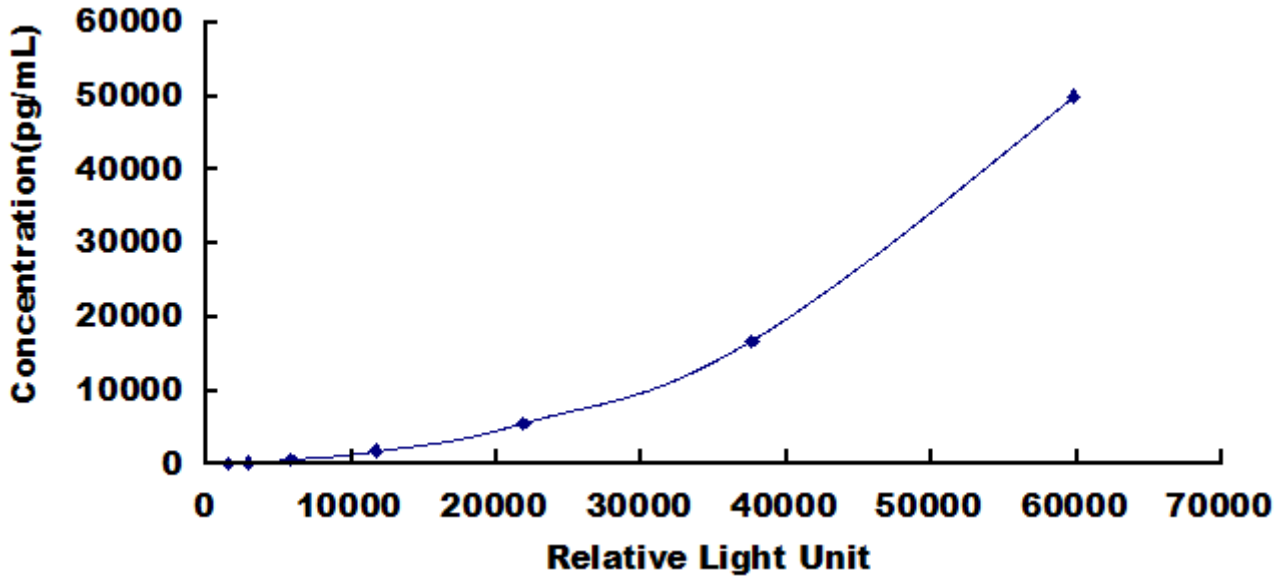
人甲胎蛋白 (αFP) 检测试剂盒标准曲线
