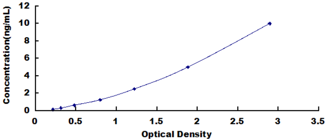
人低氧上调节因子 1 (HYOU1) 检测试剂盒标准曲线
