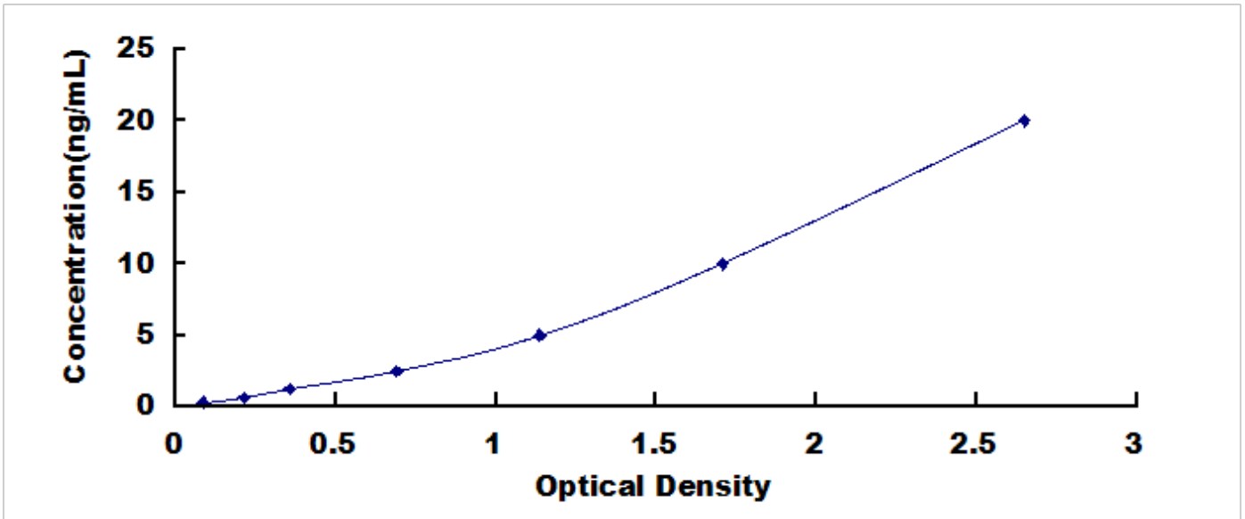
大鼠 3-羟基 3-甲基戊二酰辅酶 A 还原酶 (HMGCR) 检测试剂盒标准曲线
