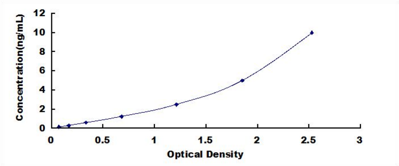
人激活素 A 受体 I (ACVR1) 检测试剂盒标准曲线
