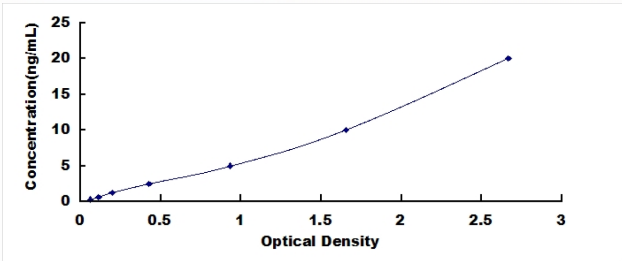
兔脂联素 (ADPN) 检测试剂盒标准曲线
