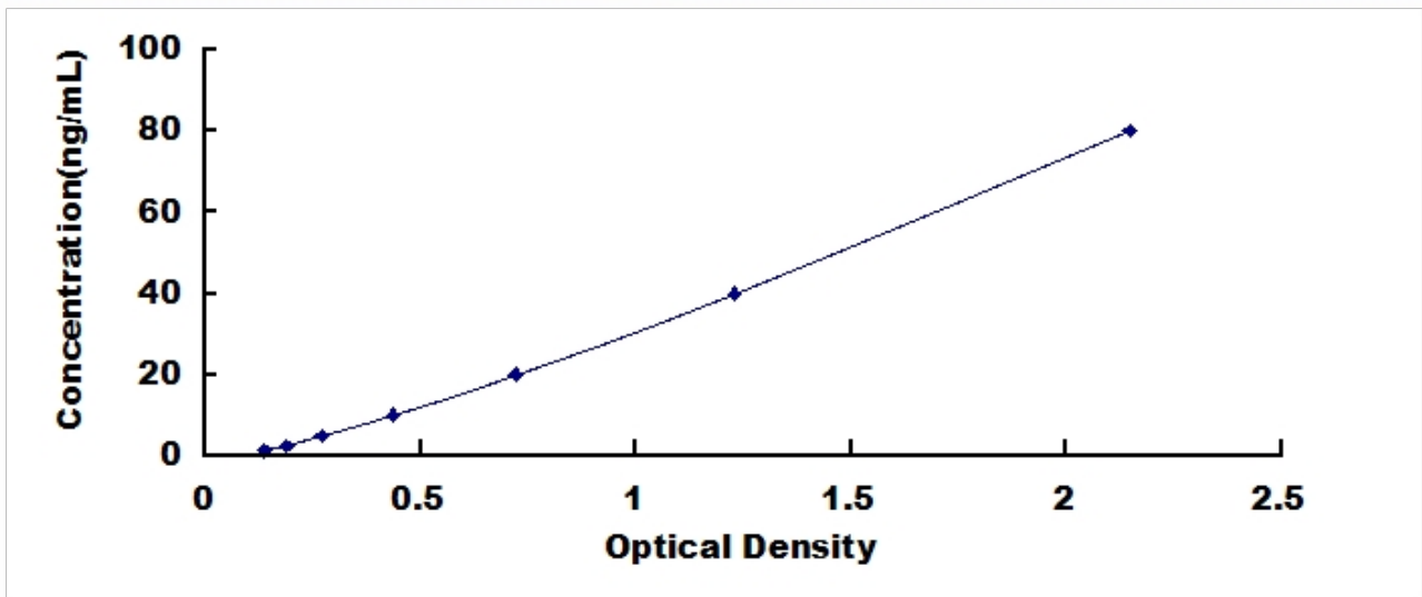
小鼠锌结合 α 2-糖蛋白 1 (aZGP1) 检测试剂盒标准曲线
