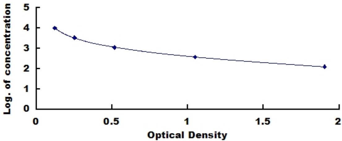
恒河猴 C-肽(CP)检测试剂盒标准曲线
