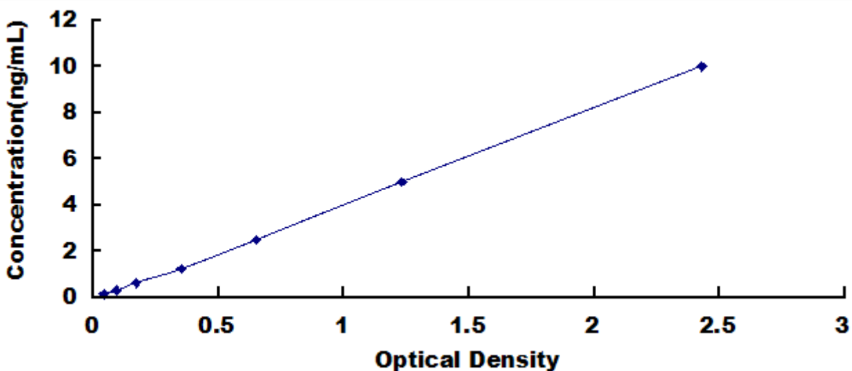
大鼠纤溶抑制因子(TAFI)检测试剂盒标准曲线
