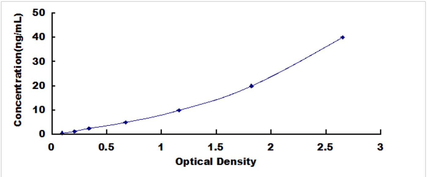
人羧肽酶 E (CPE) 检测试剂盒标准曲线
