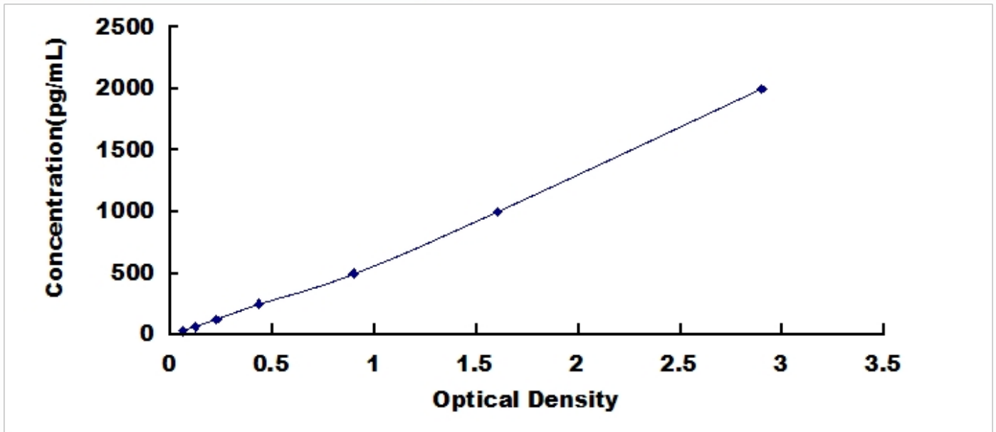
人趋化因子 C-C-基元受体 3 (CCR3) 检测试剂盒标准曲线
