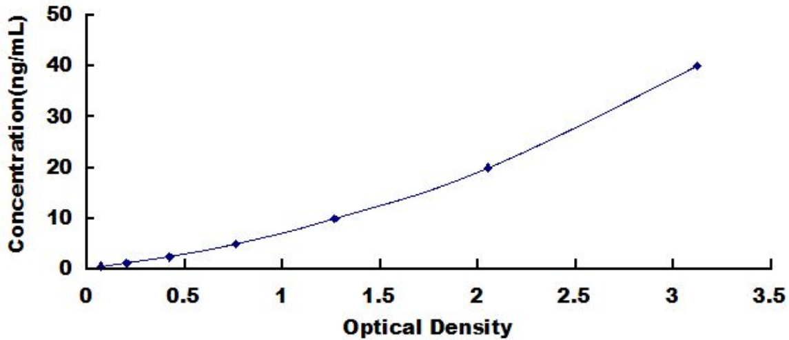
人III型胶原 α 1 (COL3 α 1) 检测试剂盒标准曲线
