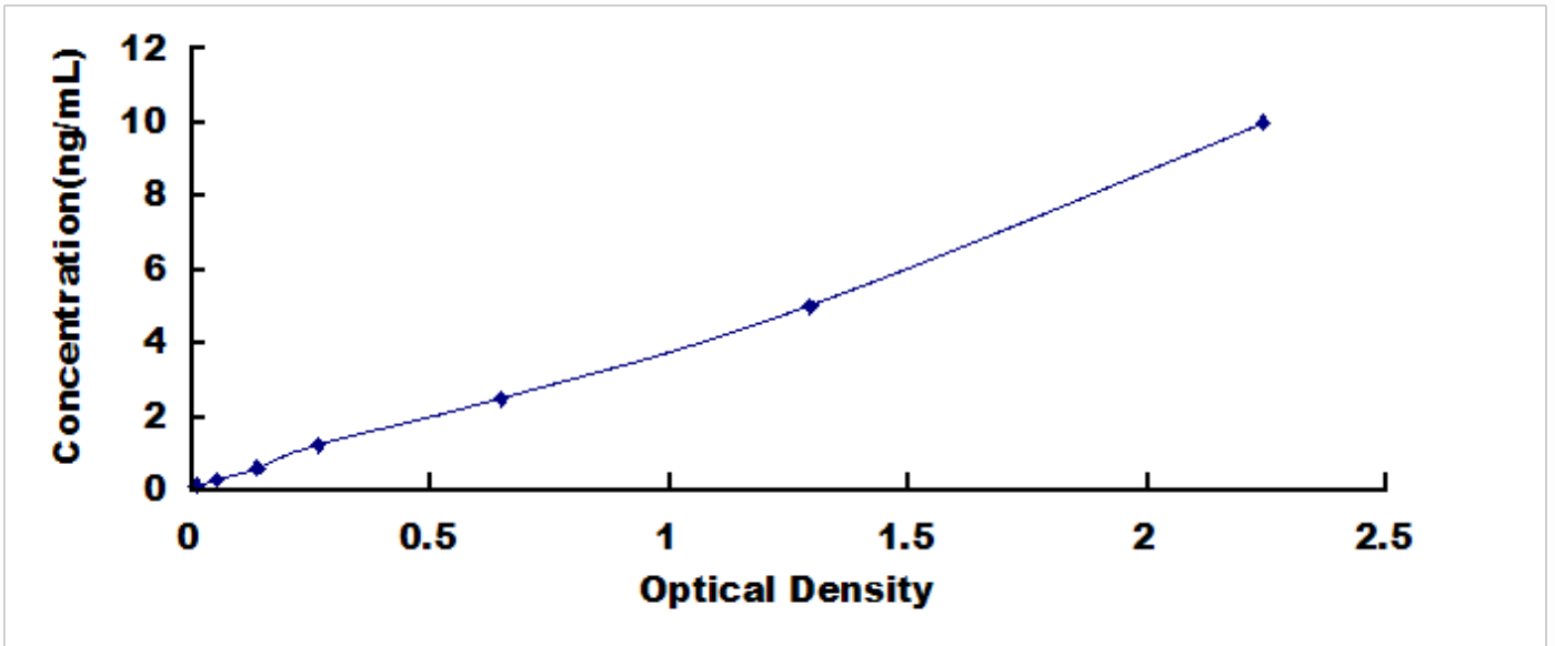
人冠蛋白 1A(CORO1A) 检测试剂盒标准曲线
