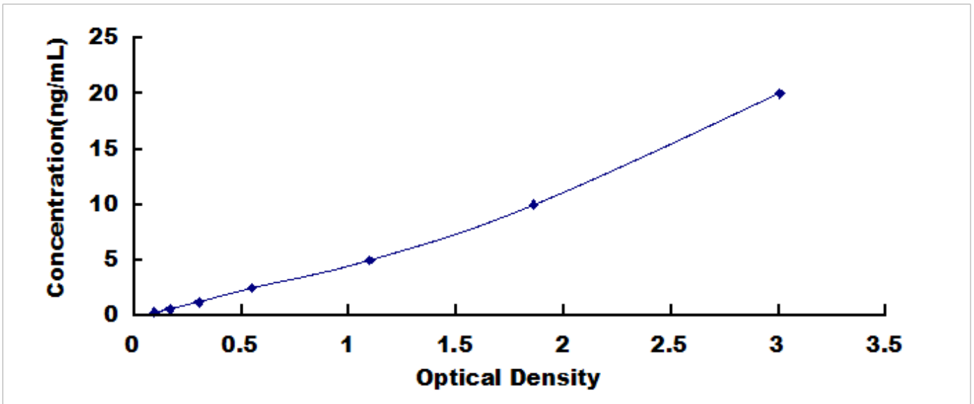
小鼠晶状体蛋白 \beta A1 (CRY \beta A1) 检测试剂盒标准曲线
