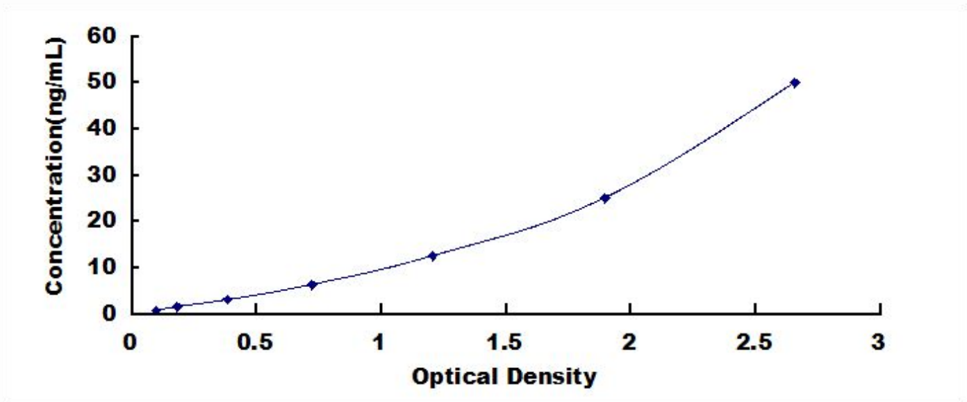
人细胞色素 P450 家族成员 2E1 (CYP2E1) 检测试剂盒标准曲线
