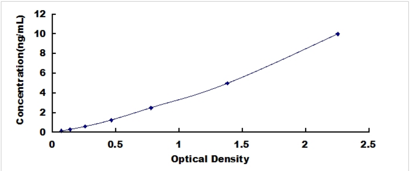
人二甲基精氨酸二甲胺水解酶 1 (DDAH1) 检测试剂盒标准曲线
