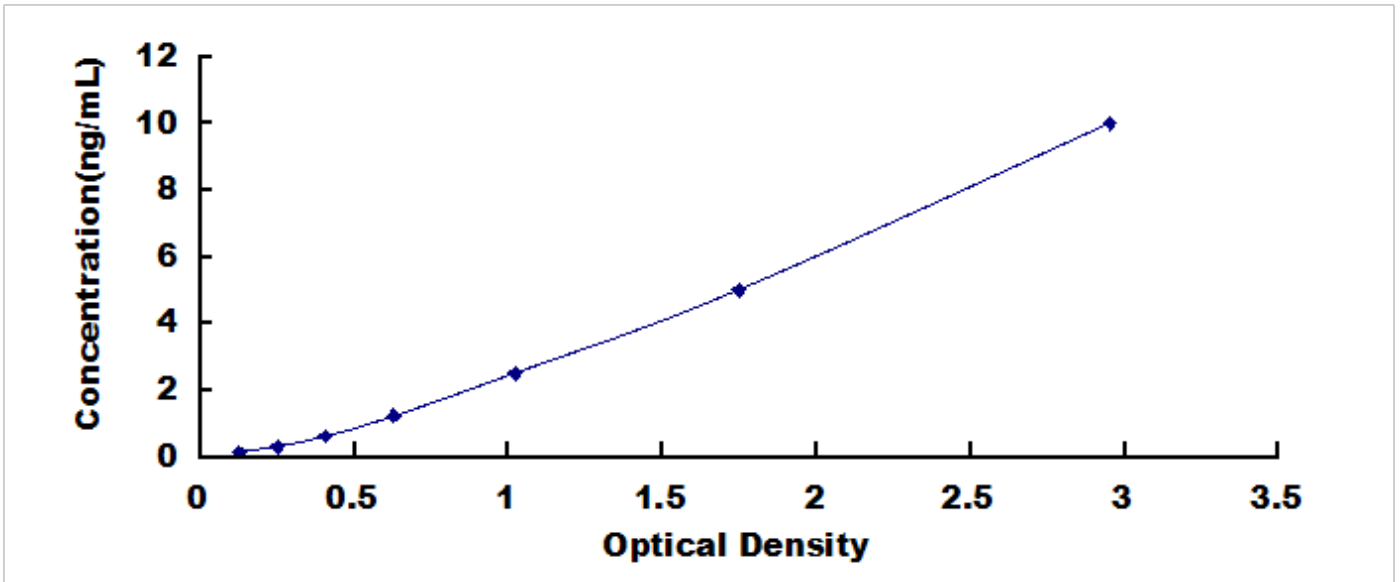
人延伸因子极长链脂肪酸样蛋白 1 (ELOVL1) 检测试剂盒标准曲线
