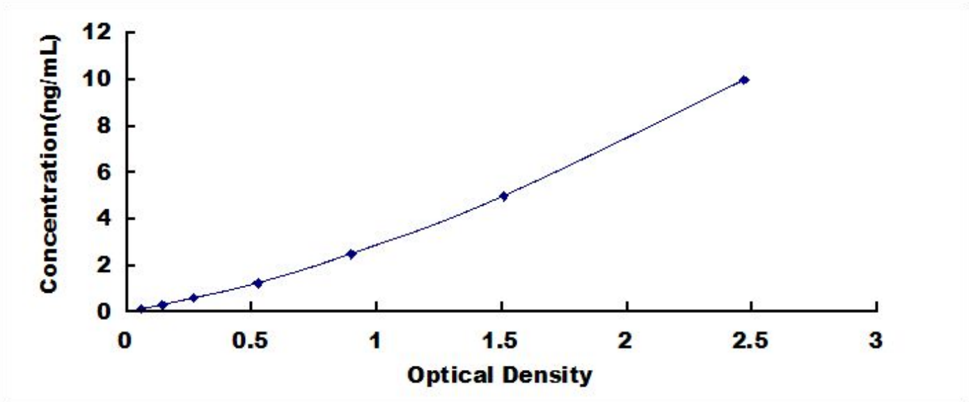
人 Enah/Vasp 样蛋白 (EVL) 检测试剂盒标准曲线
