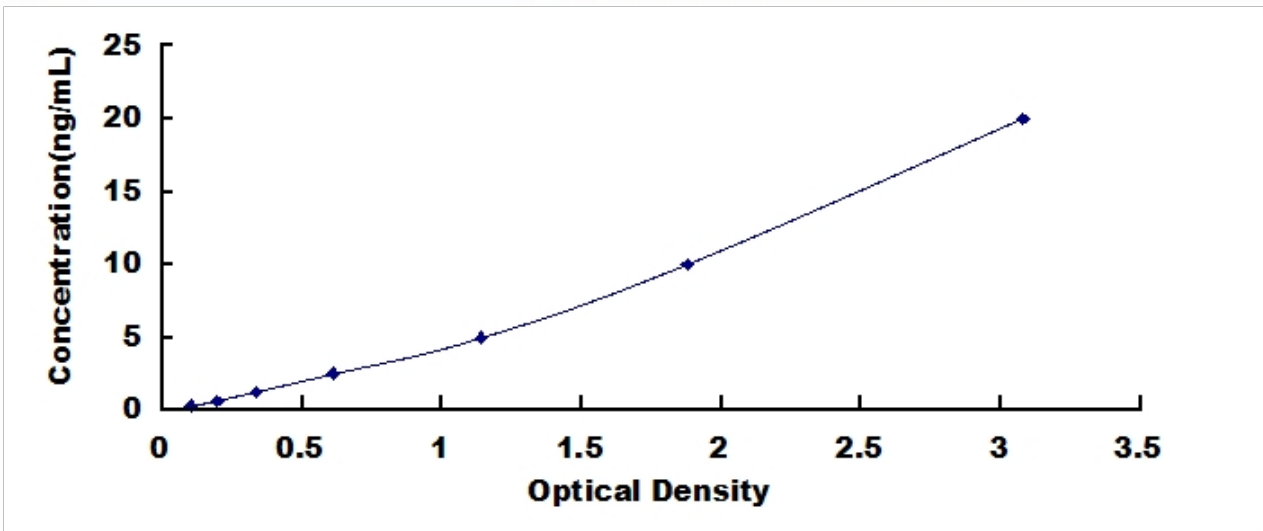
猪肝型脂肪酸结合蛋白 (FABP1) 检测试剂盒标准曲线
