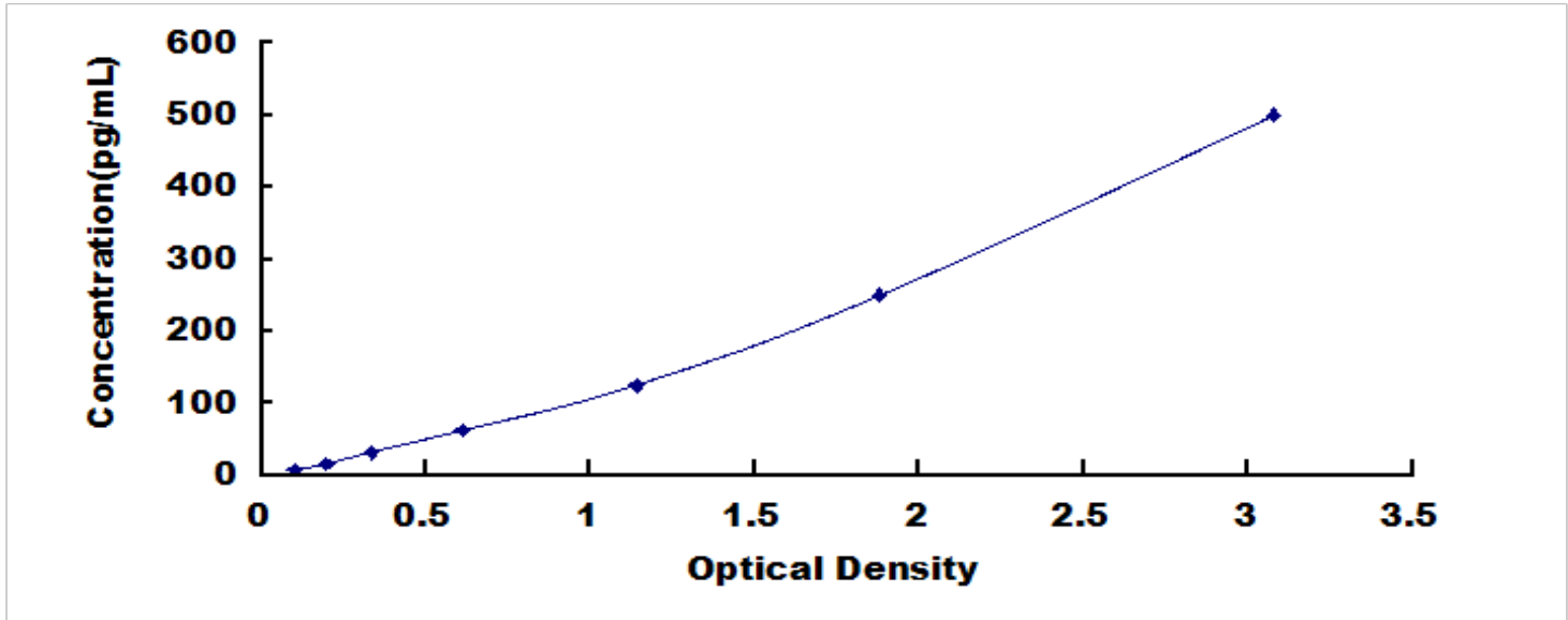
小鼠成纤维细胞生长因子 23 (FGF23) 检测试剂盒标准曲线
