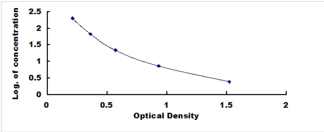
恒河猴促卵泡素 (FSH) 检测试剂盒标准曲线
