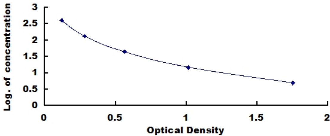
\gamma -氨基丁酸( \gamma ABA)检测试剂盒标准曲线
