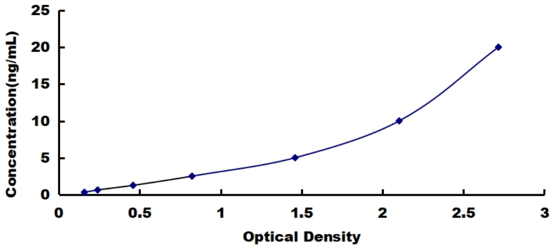
大鼠糖皮质激素受体 \alpha (GR \alpha ) 试剂盒标准曲线
