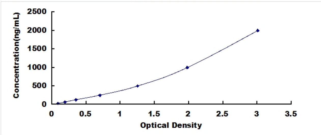
小鼠结合珠蛋白(Hpt)检测试剂盒标准曲线
