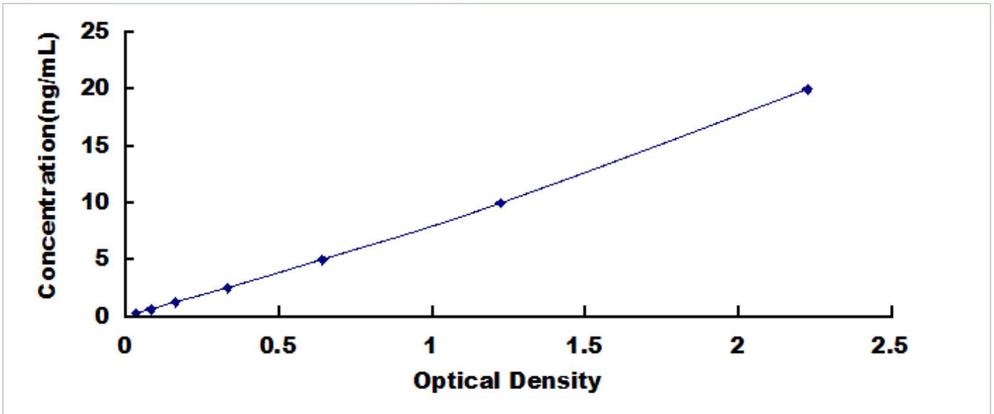
人组蛋白脱乙酰基酶 4 (HDAC4) 检测试剂盒标准曲线
