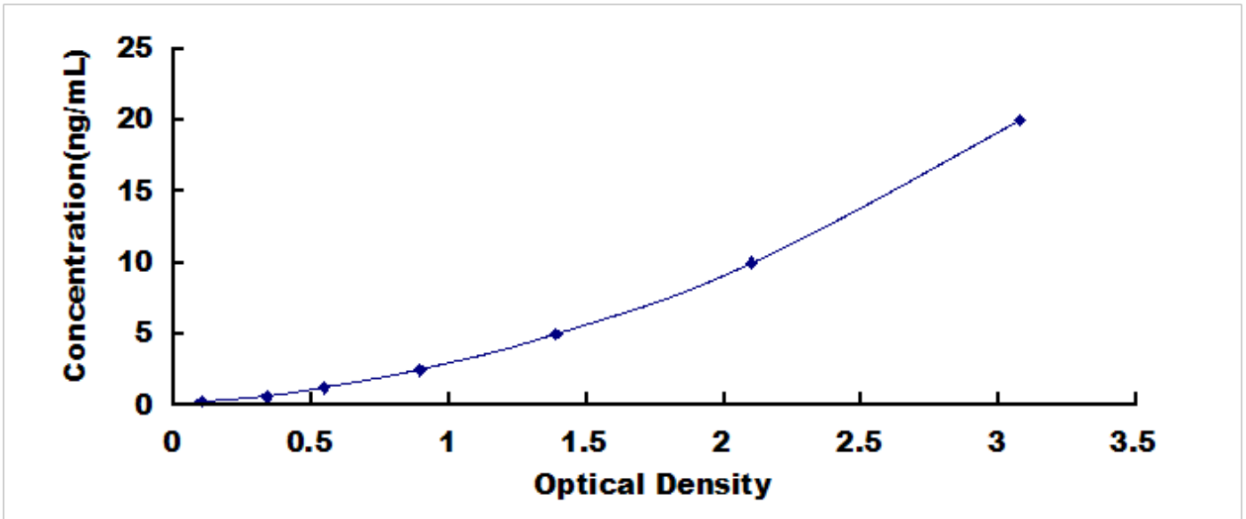
小鼠胰岛素受体底物 1 (IRS1) 检测试剂盒标准曲线
