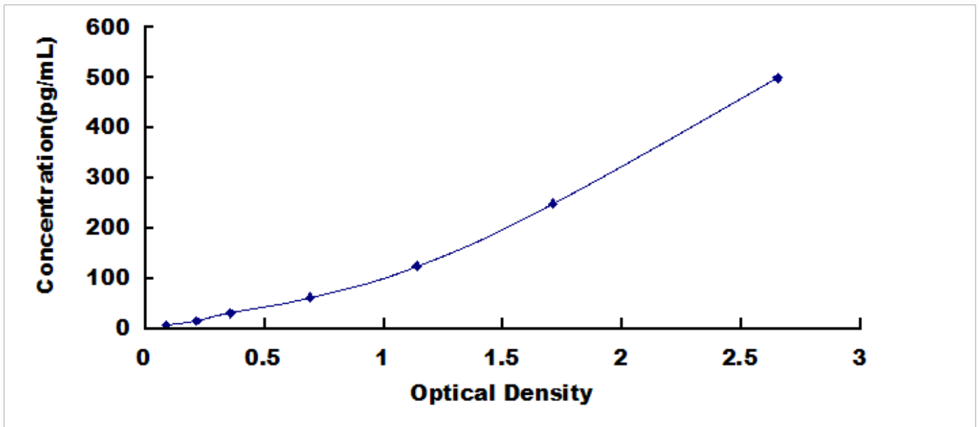
人干扰素 \alpha (IFN \alpha ) 检测试剂盒标准曲线
