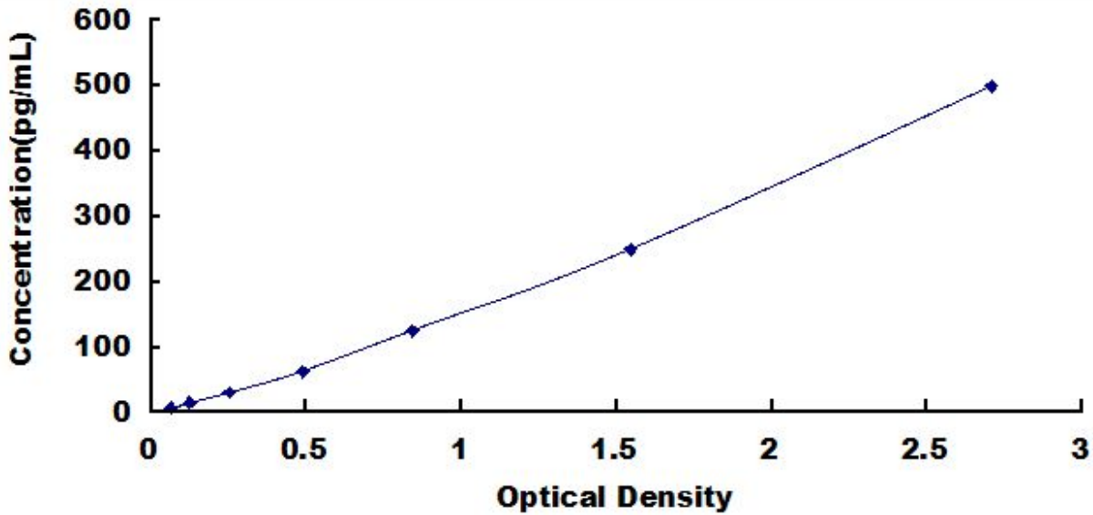
鸡白介素 1β (IL1β) 检测试剂盒标准曲线
