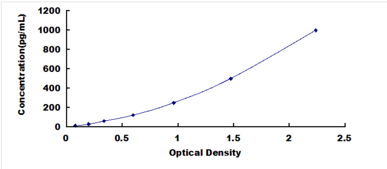
猪白介素 10(IL10) 检测试剂盒标准曲线
