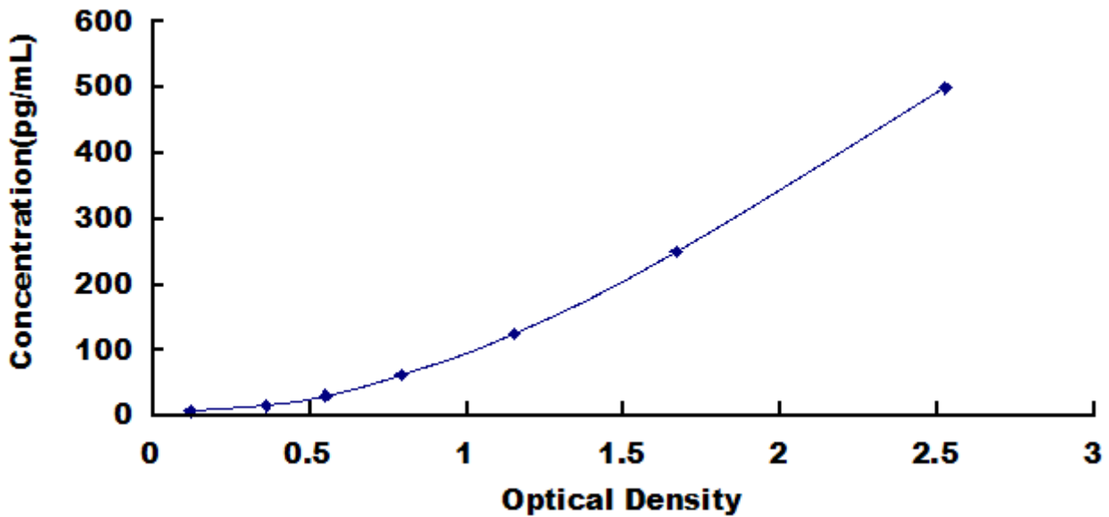
兔白介素 10(IL10)检测试剂盒标准曲线
