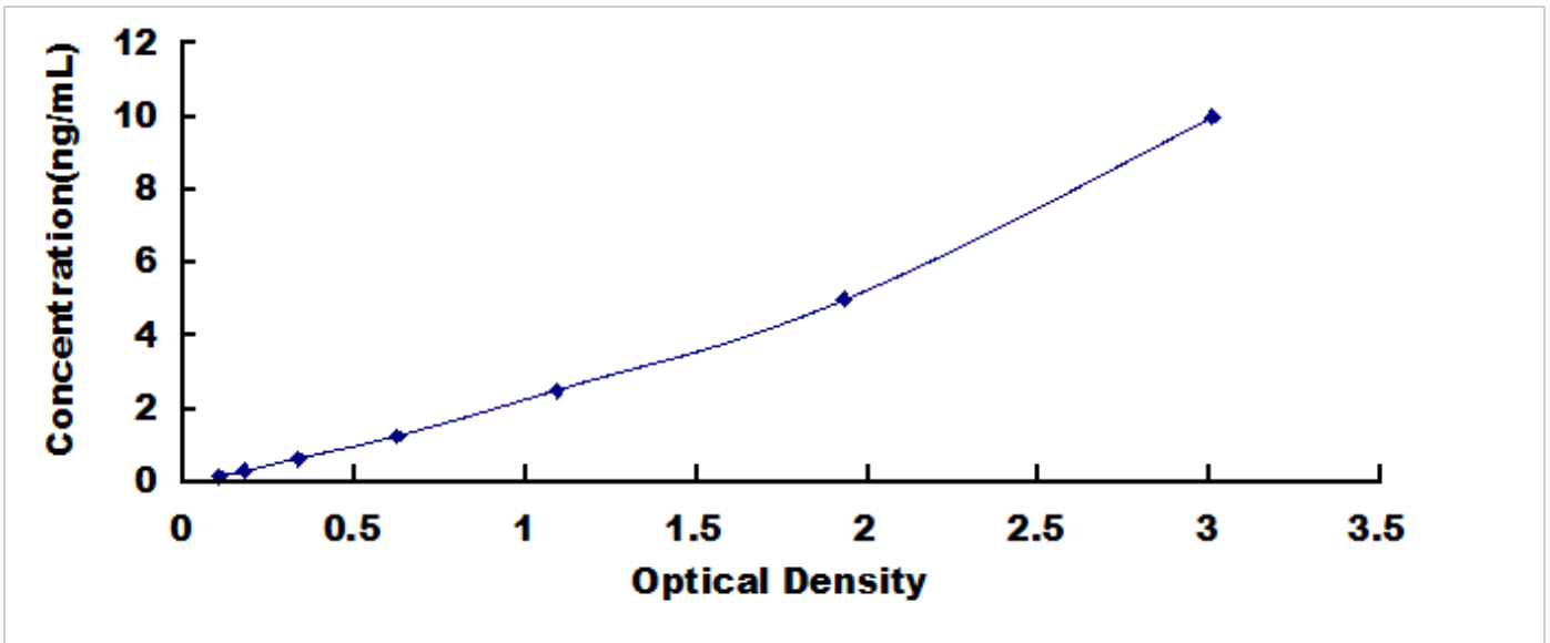
大鼠白介素 10 受体 \alpha (IL10R \alpha ) 检测试剂盒标准曲线
