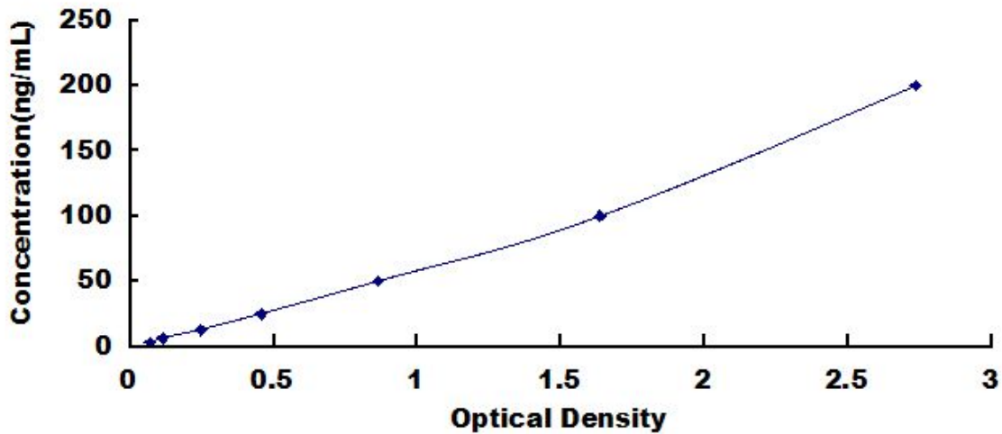
大鼠乳酸脱氢酶 C (LDHC) 检测试剂盒标准曲线
