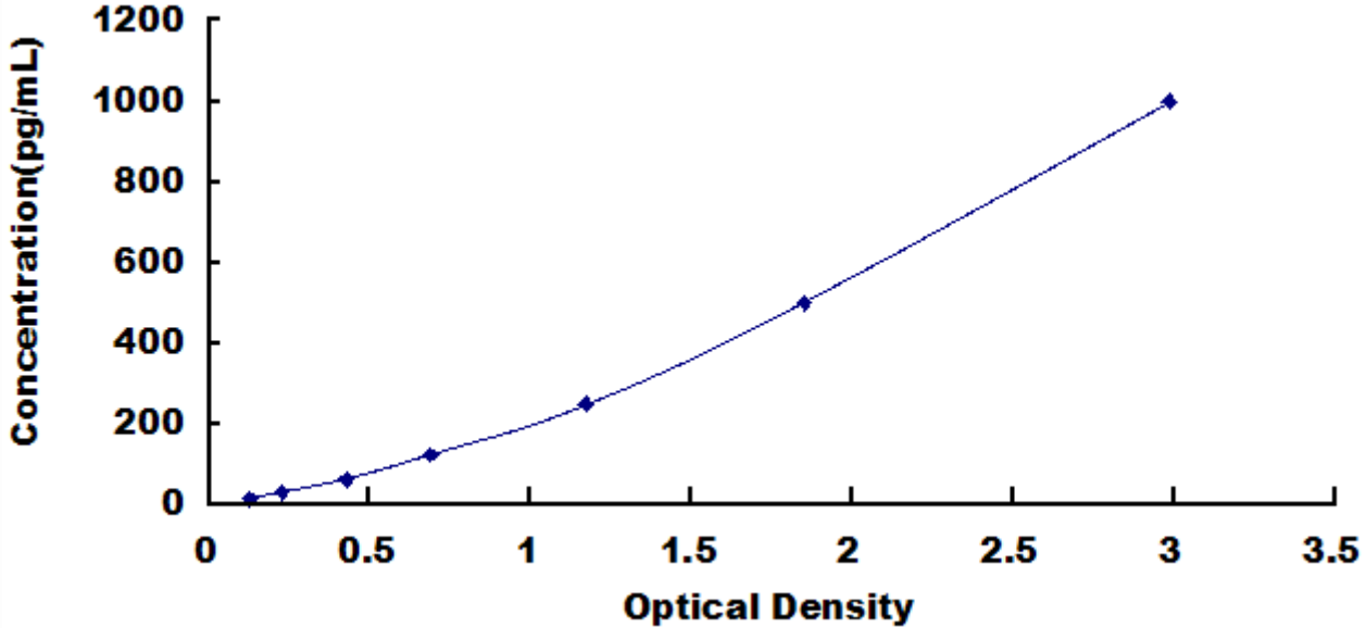
人白细胞衍生趋化因子 2 (LECT2) 检测试剂盒标准曲线
