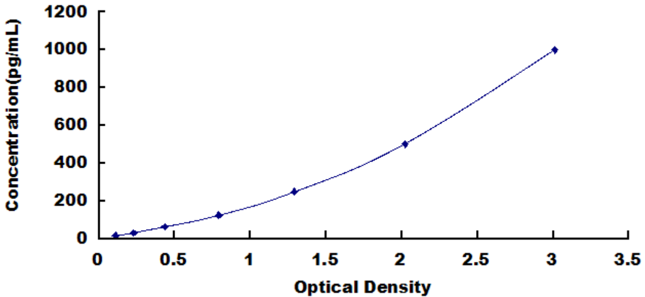
小鼠巨噬细胞炎性蛋白 3 α (MIP3 α) 检测试剂盒标准曲线
