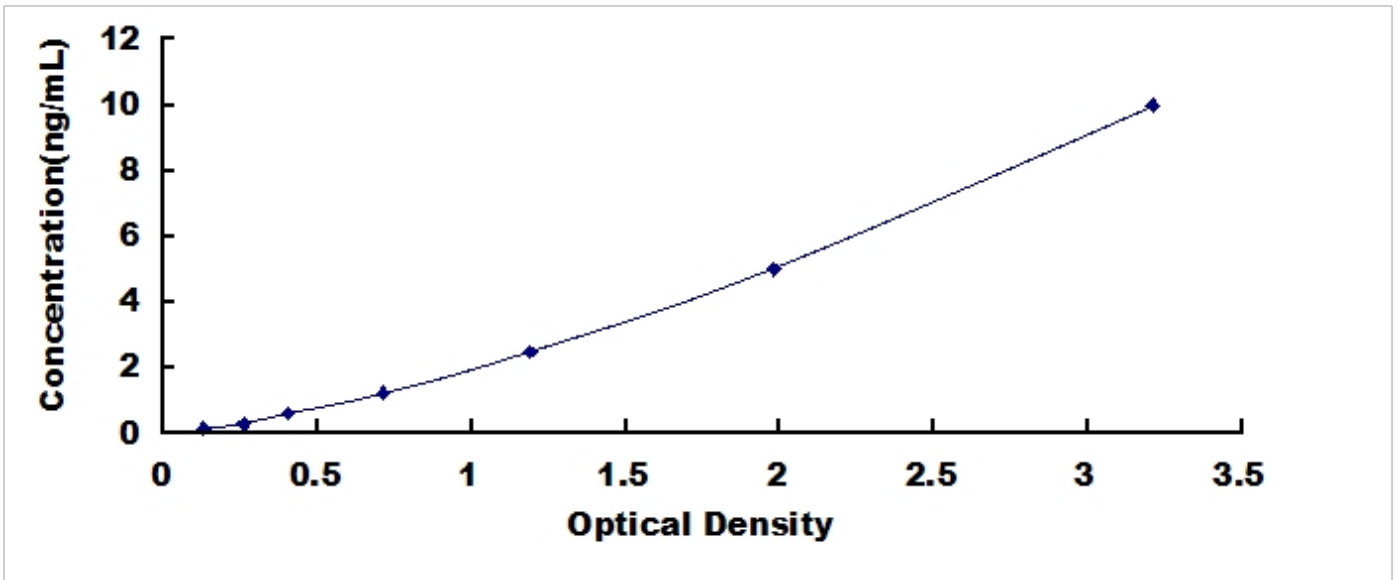
人中期因子(MK)检测试剂盒标准曲线
