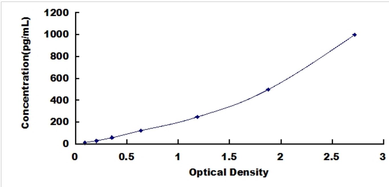
小鼠乳脂球表皮生长因子 8 (MFGE8) 检测试剂盒标准曲线
