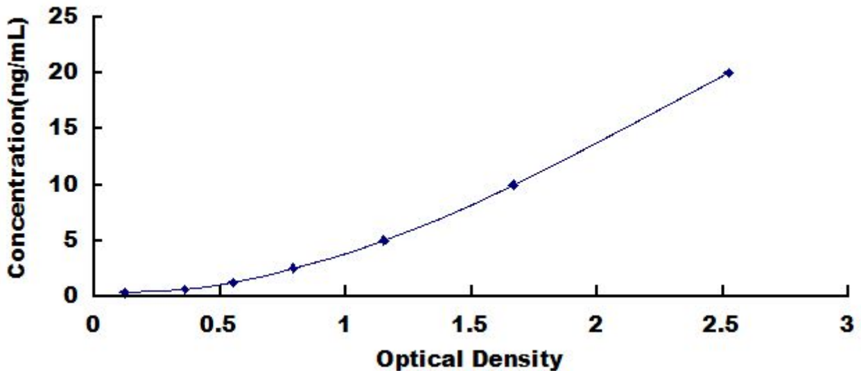
人粘蛋白 4 (MUC4) 检测试剂盒标准曲线
