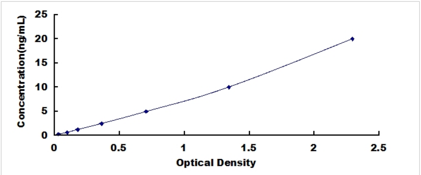
人醌 NADH 脱氢酶 1 (NQ01) 检测试剂盒标准曲线
