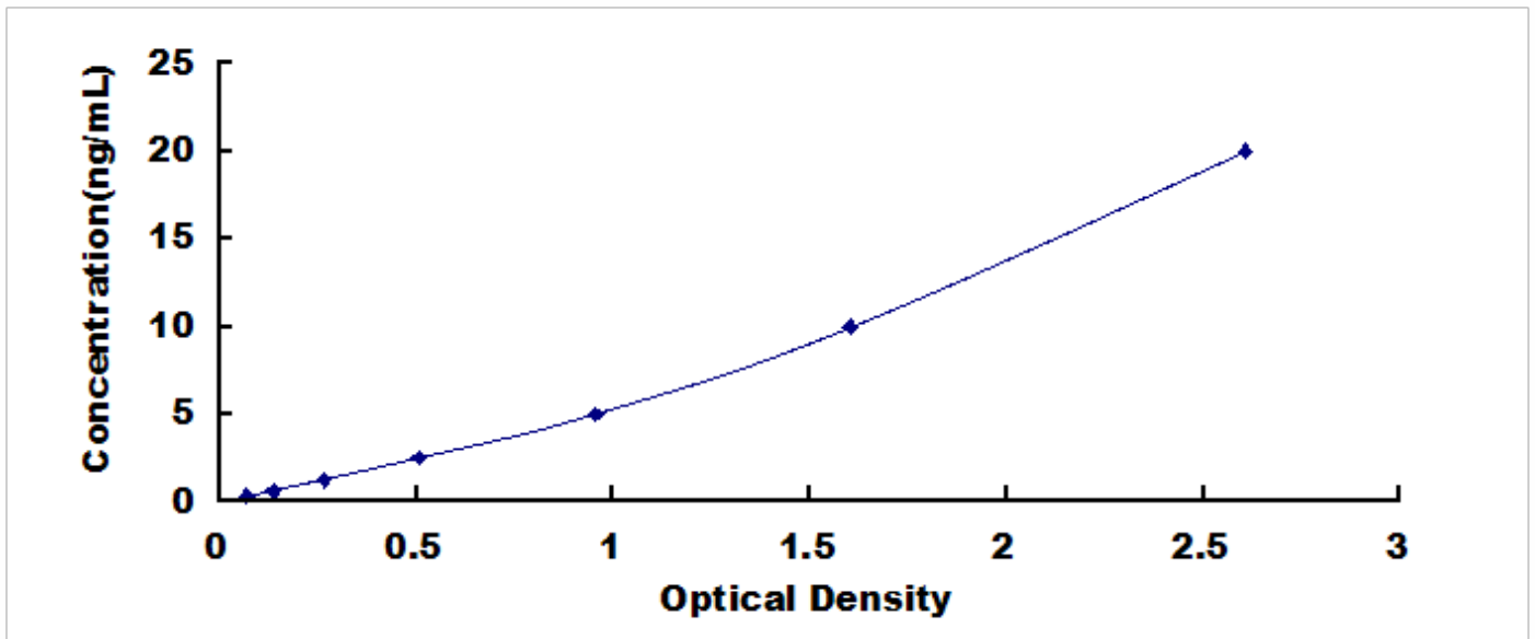
人利钠肽受体 1 (NPR1) 检测试剂盒标准曲线
