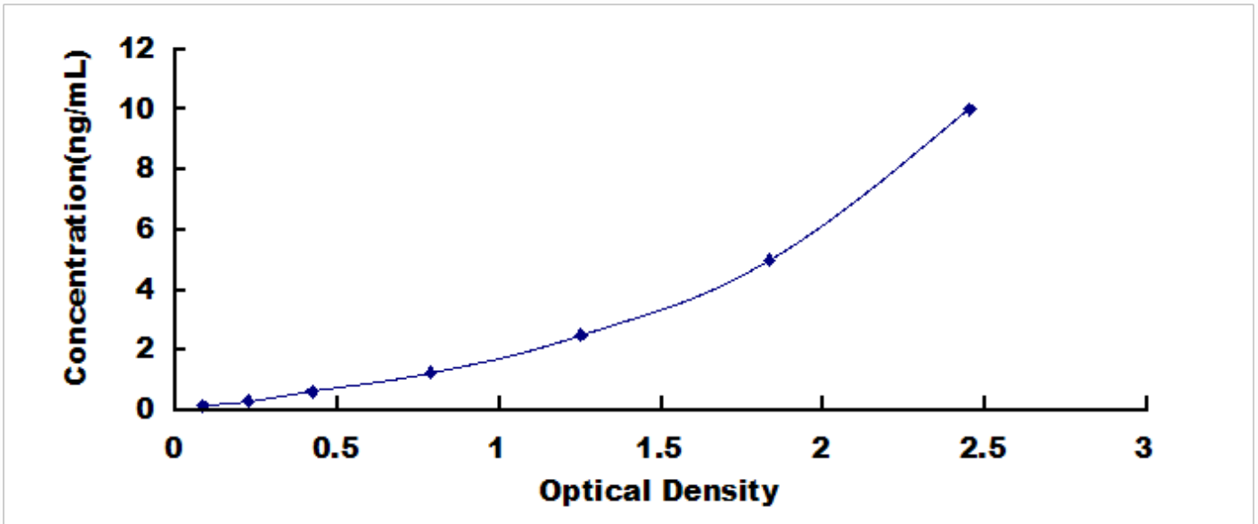
人神经调节素 1 (NRG1) 检测试剂盒标准曲线
