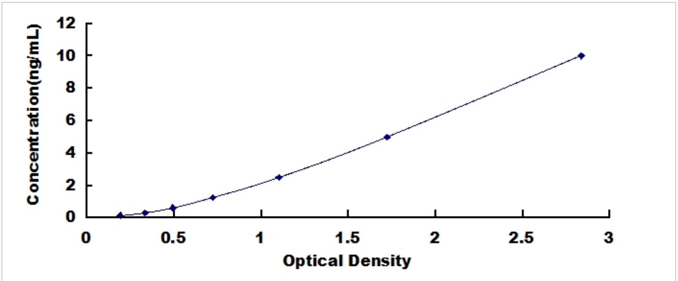
小鼠核因子 \kappa B (NF \kappa B) 检测试剂盒标准曲线
