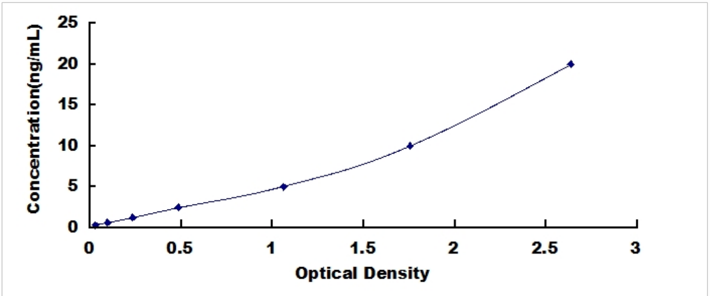
人血小板型磷酸果糖激酶(PFKP)检测试剂盒标准曲线
