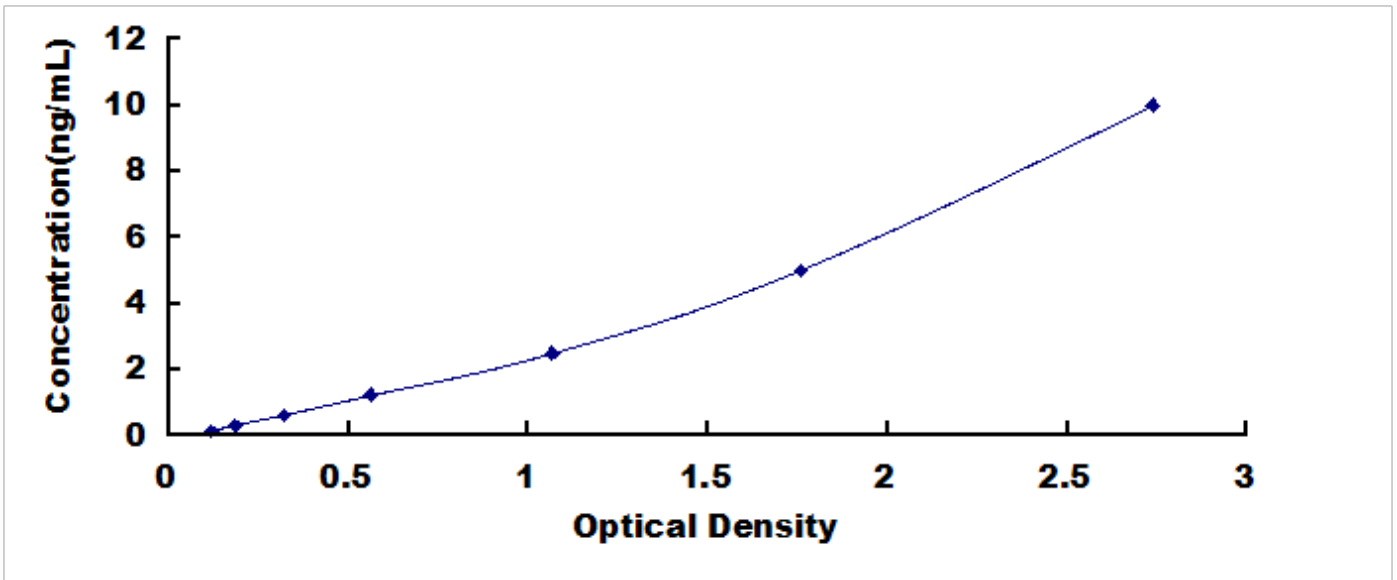
人血小板衍生生长因子受体 \alpha (PDGFR \alpha ) 检测试剂盒标准曲线
