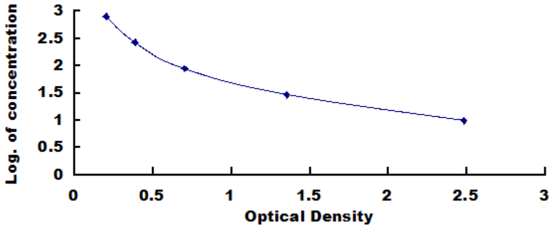
前列腺素 F2 α (PGF2 α) 检测试剂盒标准曲线
