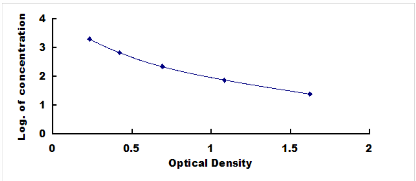
牛松弛肽 (RLN) 检测试剂盒标准曲线
