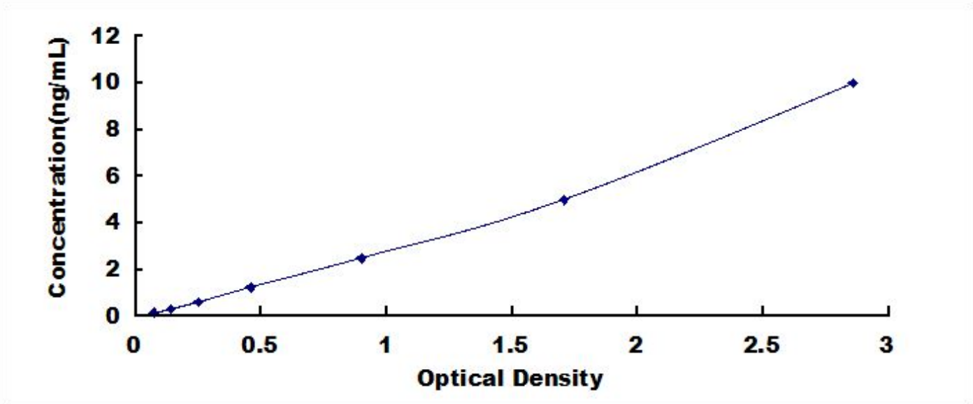
人核糖体蛋白 L6 (RPL6) 检测试剂盒标准曲线
