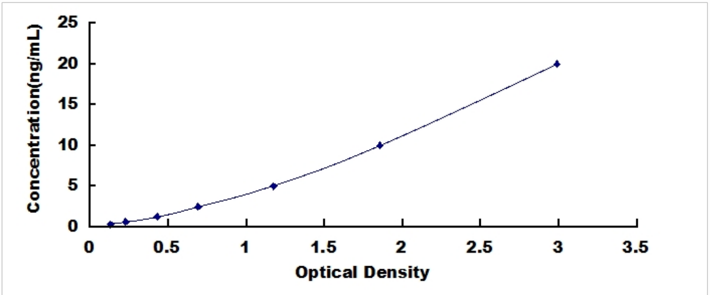
人琥珀酸脱氢酶复合体 C 亚基(SDHC)检测试剂盒标准曲线
