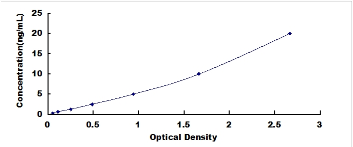
人突触囊泡蛋白 VII (SYT7) 检测试剂盒标准曲线
