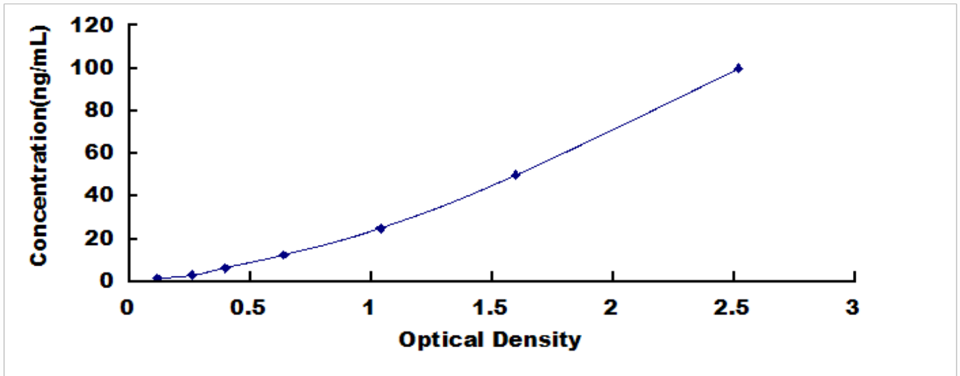
大鼠多配体蛋白聚糖 1 (SDC1) 检测试剂盒标准曲线
